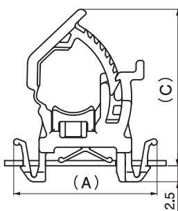
【板金実装時 (最大径)】
