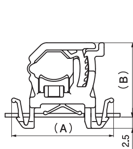
【板金実装時 (最小径)】
