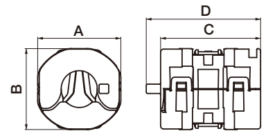
※NFT-13SB-20DKはバンド固定部付き *NFT-13SB-20DK have a band fixing part.
