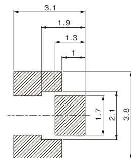
ランド寸法図 Land dimensions
