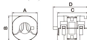
※NFT-13S, 14Nはバンド固定部付き *NFT-13S, NFT-14N have a band fixing part.
